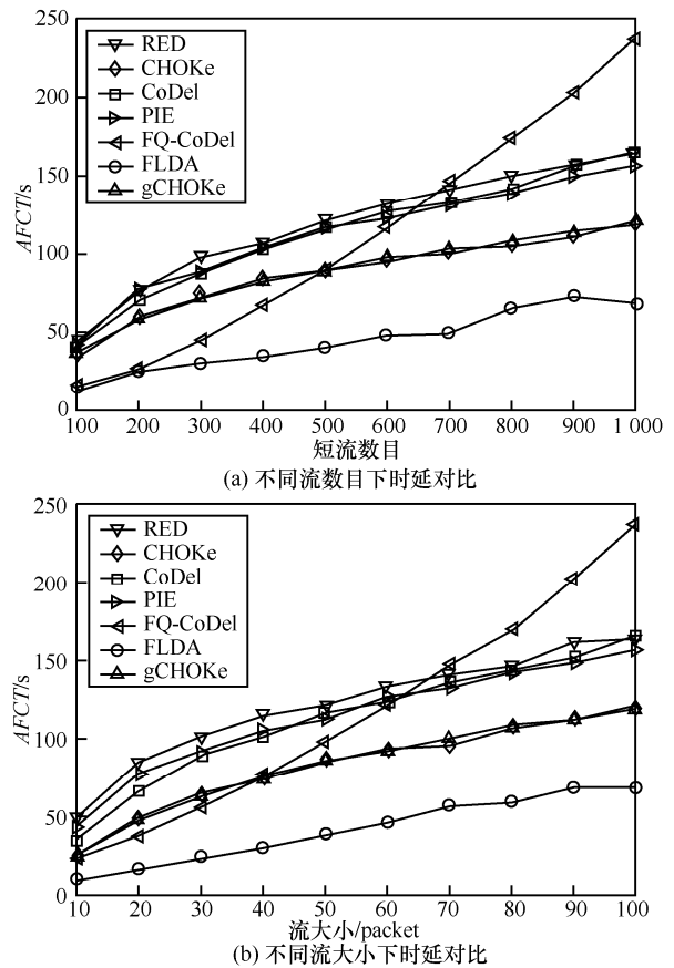
图 8 多瓶颈链路实验中的时延对比
