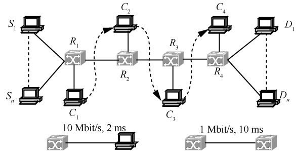
图 7 Parking-lot 多瓶颈链路实验拓扑
